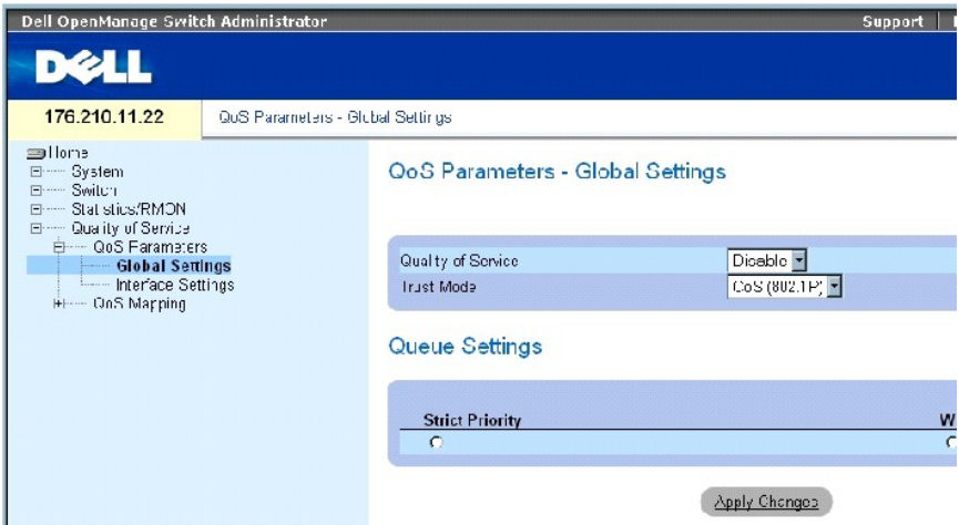
그림 9-1. 전역 설정
