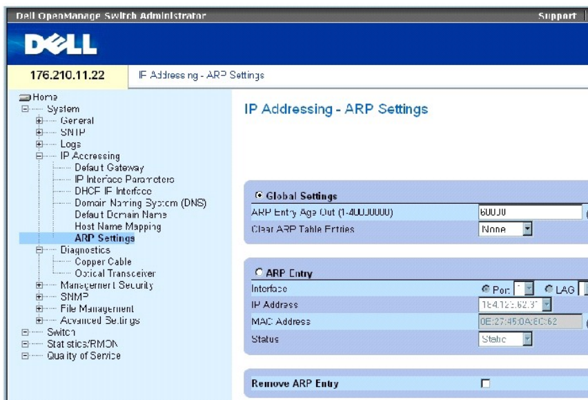
그림 6-35. ARP 설정
