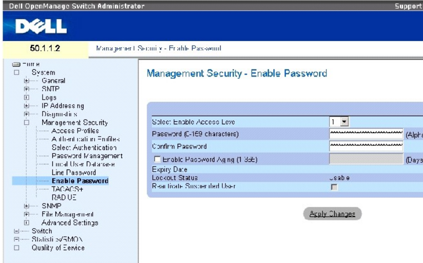
그림 6-50. 활성 암호
