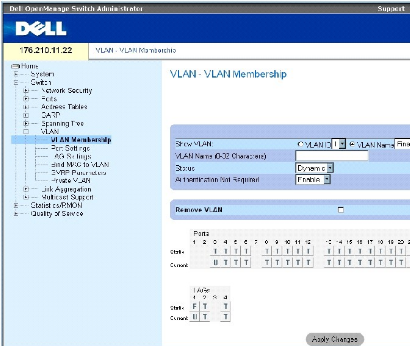
그림 7-30. VLAN 멤버십
