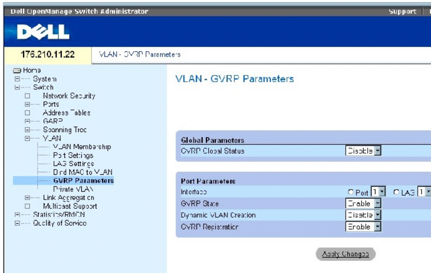
그림 7-34. GVRP 매개변수
