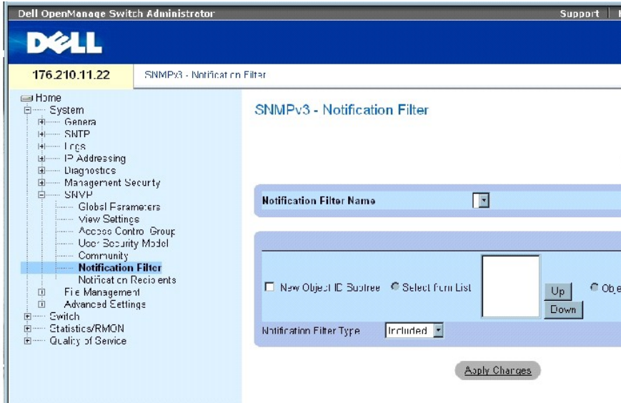
그림 6-69. 알림 필터
